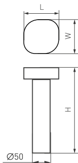
Рис. 1. Чертеж и габаритные размеры
